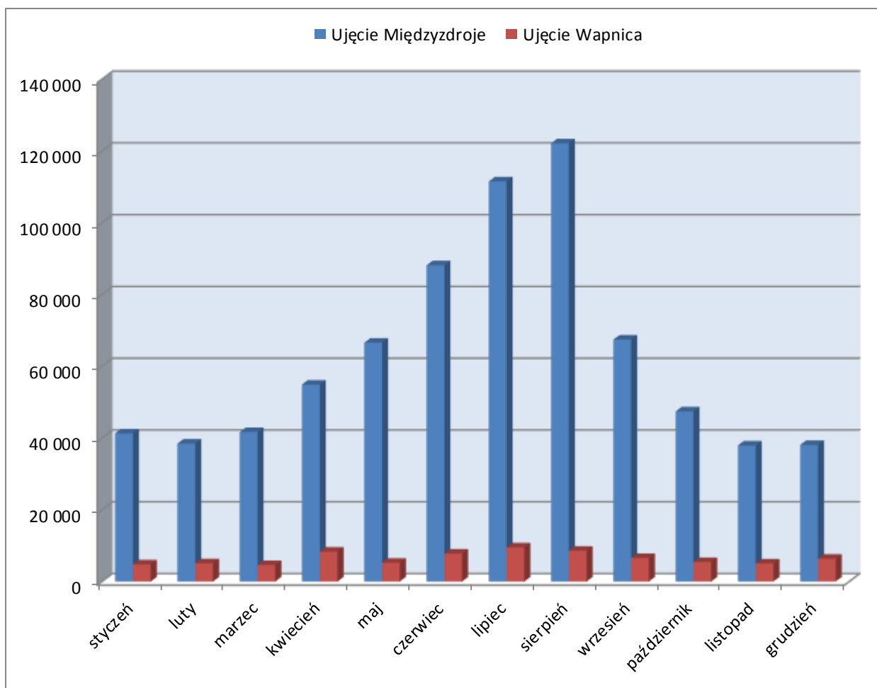
Ilustracja nr 15 - Produkcja wody w roku 2019 w poszczególnych miesiącach z dwóch ujęć – źródło własne
